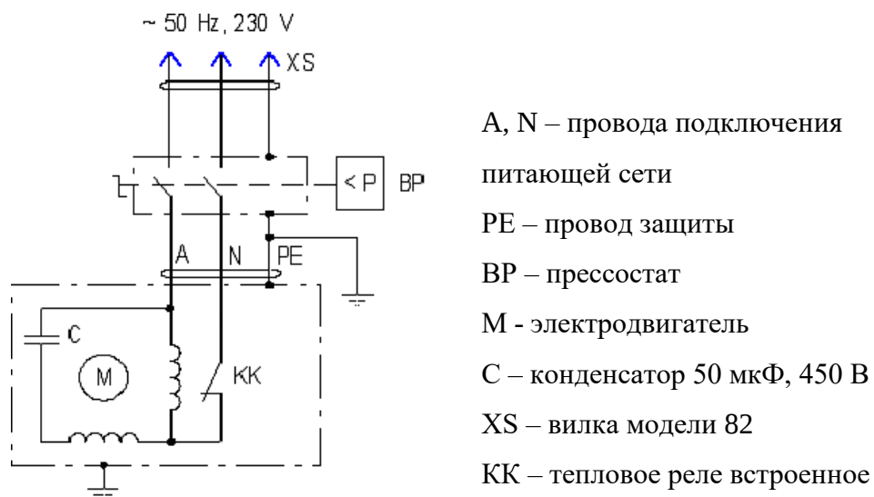
Рисунок А.1 - Схема электрическая принципиальная компрессора
