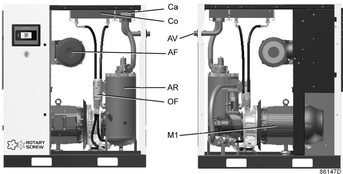
Основные компоненты
