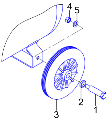
1 - Болт 2 - Шайба 3 - Колесо
