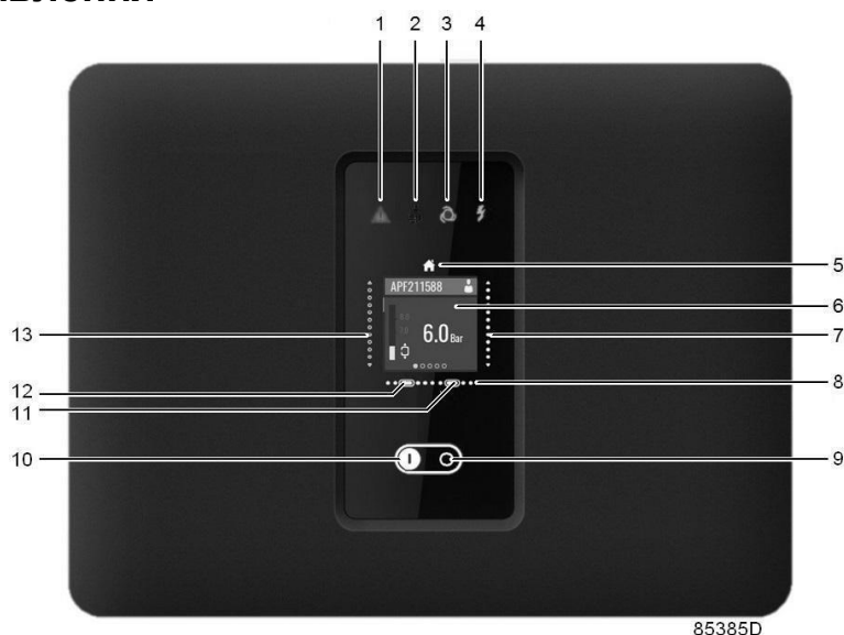
Панель управления
